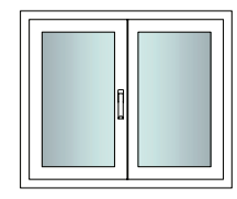
MH-DF Wandstärke: 15mm Maße: 110x92cm
