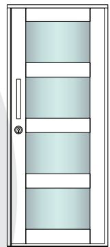
MH-ST-S Wandstärke: 15 mm Maße: 84x200cm
