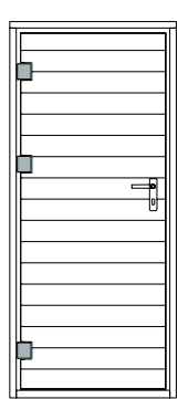
MH-ET-GG-WB Wandstärke: 15mm Maße: 84x194cm
