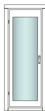
F45-K80 Wandstärke: 45mm Maße: 80x40cm
