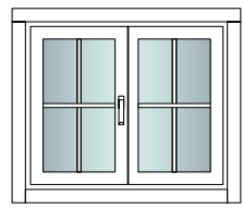
F28-DF Wandstärke: 28mm Maße: 110x92cm
