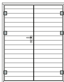
MH-DT-GG-WB Grubość ściany (profilu): 15mm Wymiary: 150x194cm
