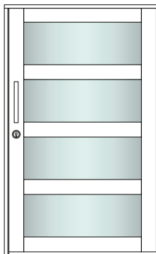
NH-ST-B Grubość ściany (profilu): 15 mm Wymiary: 125x200cm
