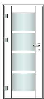
NH-ET-GV1-QS Grubość ściany (profilu): 15mm Wymiary: 84x194cm
