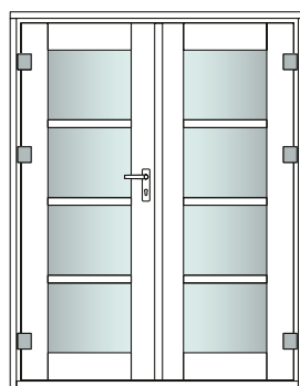
NH-DT-GV1-QS Grubość ściany (profilu): 15mm Wymiary: 150x194cm
