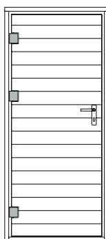
MH-ET-GG-WB Grubość ściany (profilu): 15mm Wymiary: 84x194cm
