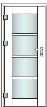
NH-ET-GV1-QS Épaisseur du mur (madrers): 15mm Dimensions (I/L): 84x194cm
